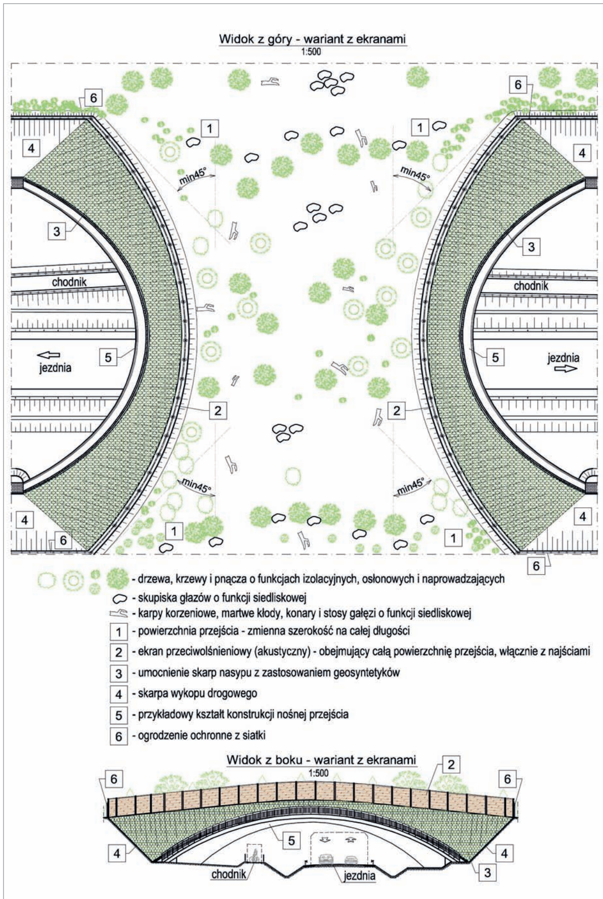
Rysunek 3. Optymalne rozwiązania projektowe przejścia górnego przy korzystnej niwielce drogi (droga w wykopie) – wariant z ekranami przegrodowymi.
