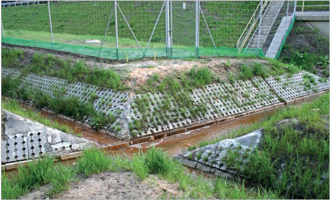
Fot. 107. Umocnione rowy przecinające strefy naprowadzania zwierząt do przejścia dolnego.
