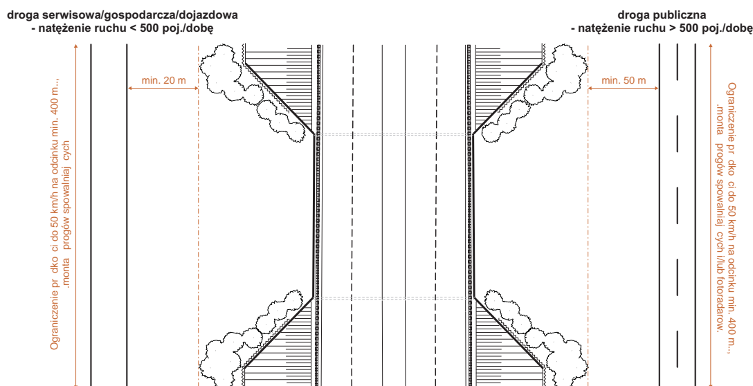
Ryc. 42. Projektowanie przejść dolnych oraz zsynchronizowanych przejść po powierzchni jezdni w przypadku równoległej drogi serwisowej (o natężeniu ruchu <math>< 500</math> poj./dobę) i publicznej (o natężeniu ruchu > 500 poj./dobę).
