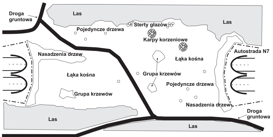
Ryc. 12. Most Asp Holz (autostrada N7, Szwajcaria) – przykład zagospodarowania powierzchni przejścia krajobrazowego w obszarze leśnym.
