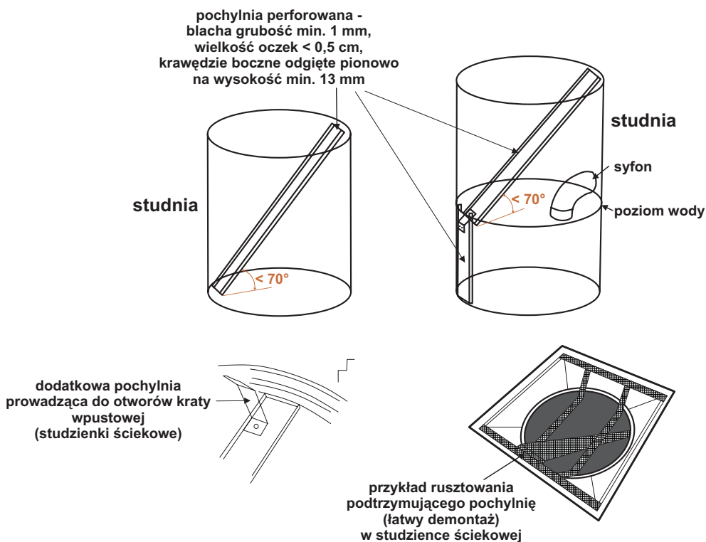
Ryc. 62. Schemat pochylni umożliwiających wychodzenie zwierząt ze studni otwartych i zamkniętych (z kratą wpadową).
