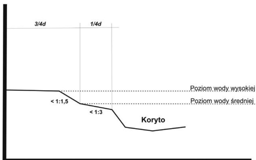
Schemat kształtowania półek ziemnych w przejściach dla zwierząt zespolonych z ciekami wodnymi
