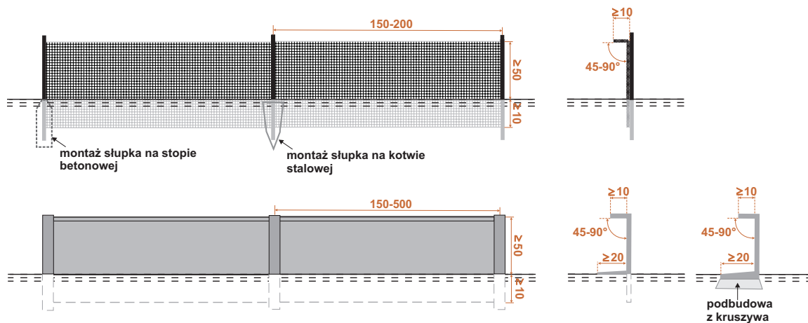
Ryc. 54. Zalecane rozwiązania i parametry kluczowych elementów ogrodzeń ochronno-naprowadzających dla małych zwierząt – wykonanych z siatek i pełnych płyt (wymiały w cm).
