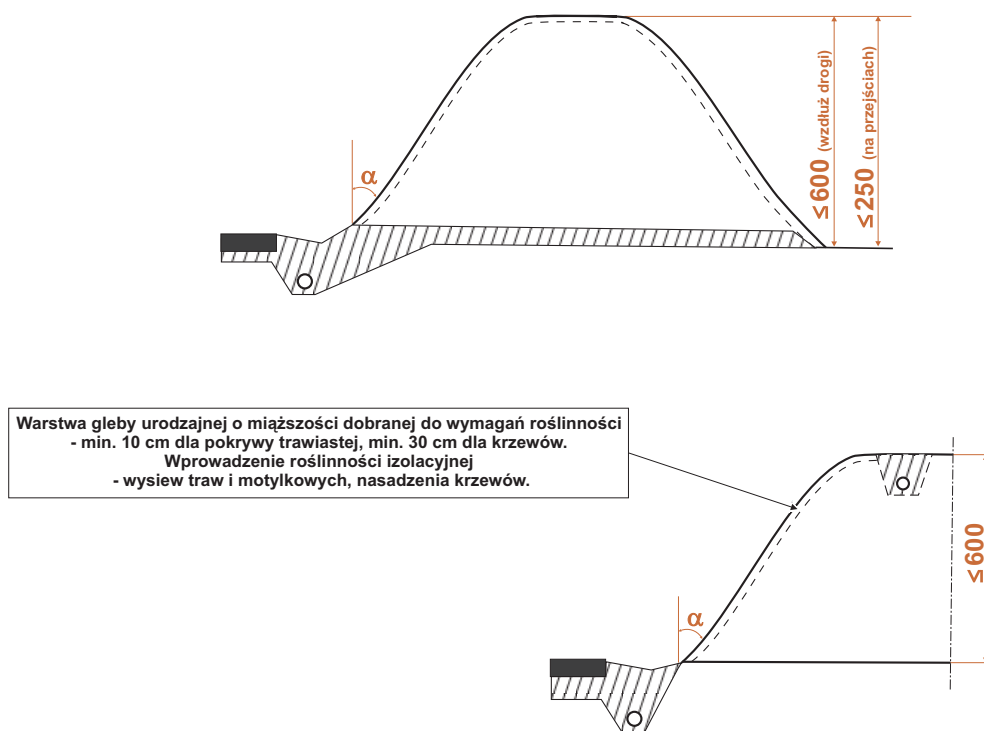
Ryc. 60. Optymalne rozwiązania ekranów ziemnych (wymiary w cm).
