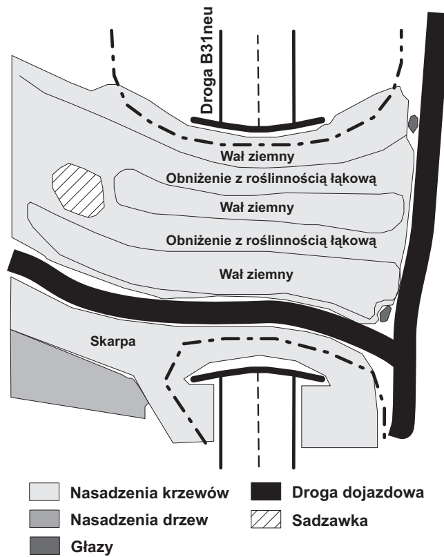
Ryc. 13. Most Schwarzgraben (droga B31neu, Niemcy) – przykład zagospodarowania powierzchni przejścia dla dużych zwierząt zespolonego z drogą lokalną w obszarze mozaiki polno-leśnej.
